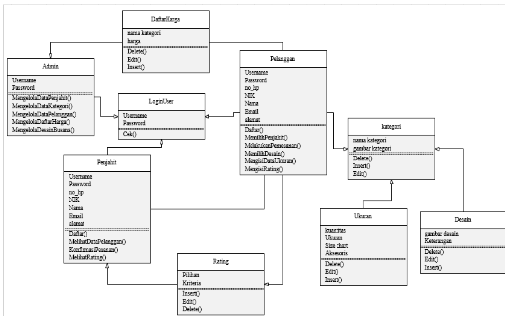
GAMBAR 5. PEMODELAN DATA
