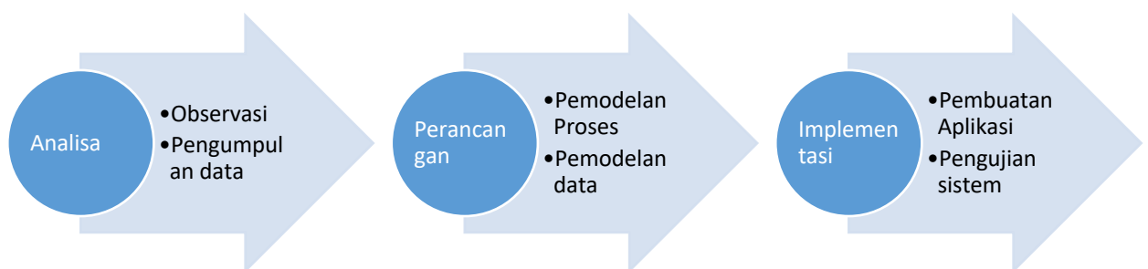
GAMBAR 1. TAHAPAN PENELITIAN
