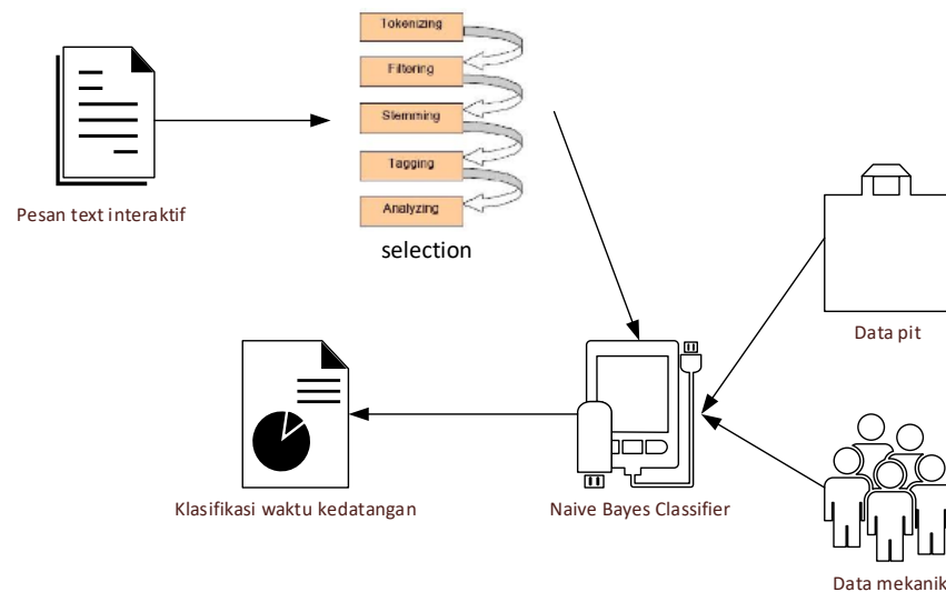
Gambar 3. Arsitektur sistem aplikasi booking servis
