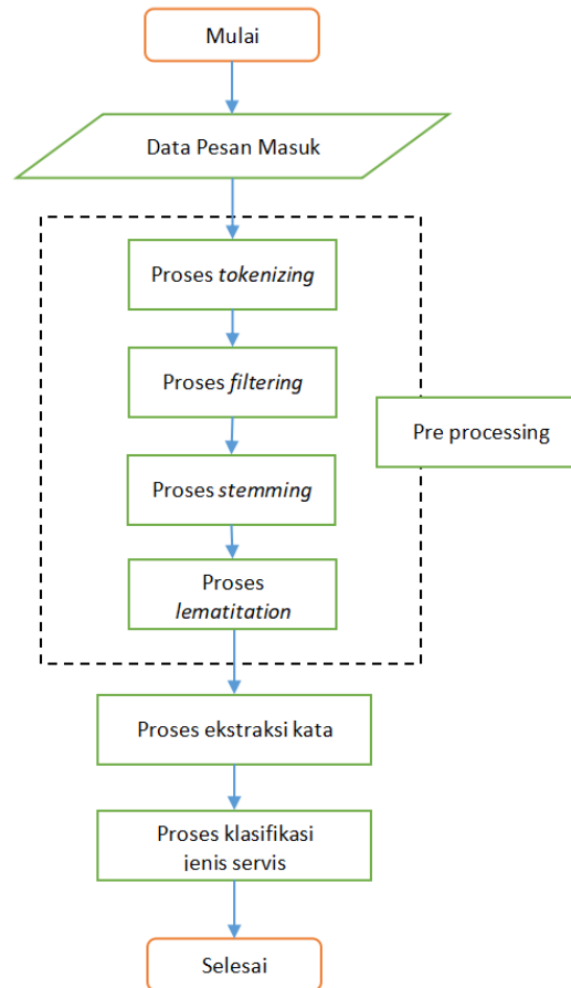
Gambar 2 Flowchart sistem yang dibangun
